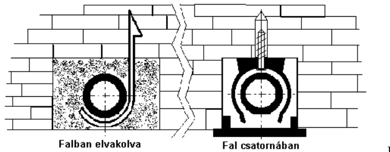
III.-14. sz. ábra A fogyasztói vezeték burkolási lehetőségei.
