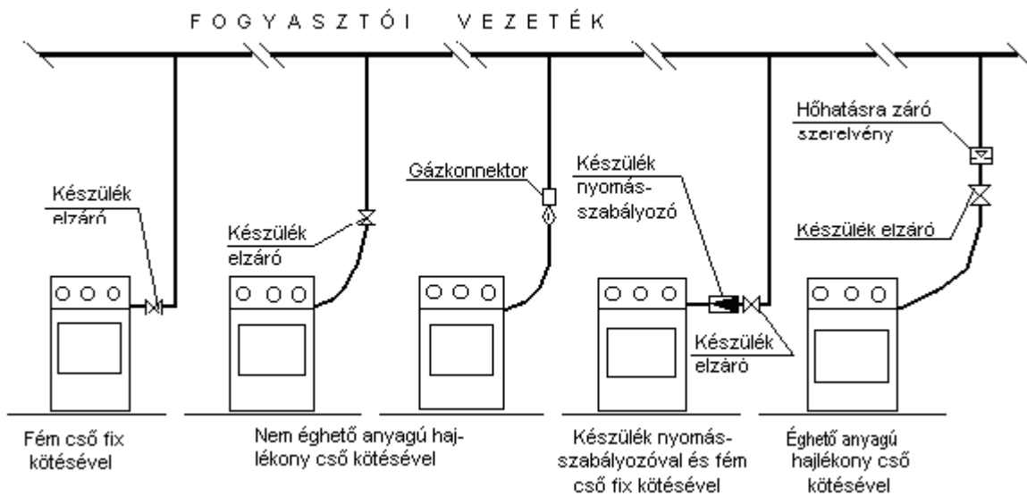
II.-6. sz. ábra Példák gázfogyasztó készülék elzáró elhelyezésére
