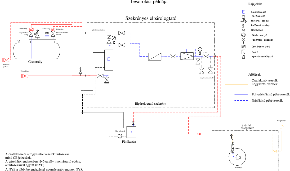
II.-10. sz. ábra A csatlakozó vezeték elpárolgatós pébégáz ellátó rendszer esetén
