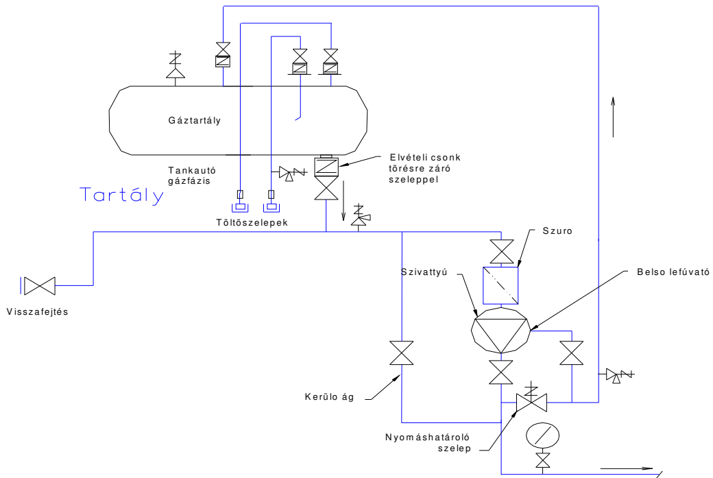
III.-12. sz. ábra Szivattyúegység elhelyezése a folyadékfázisú csatlakozó vezetékben
