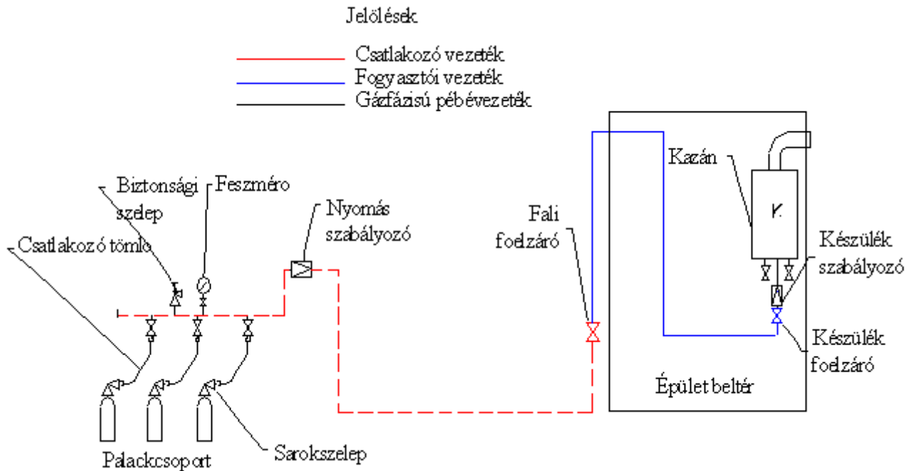
II.-12. sz. ábra Csatlakozó vezeték palackcsoportos pébégáz ellátó rendszer esetén
