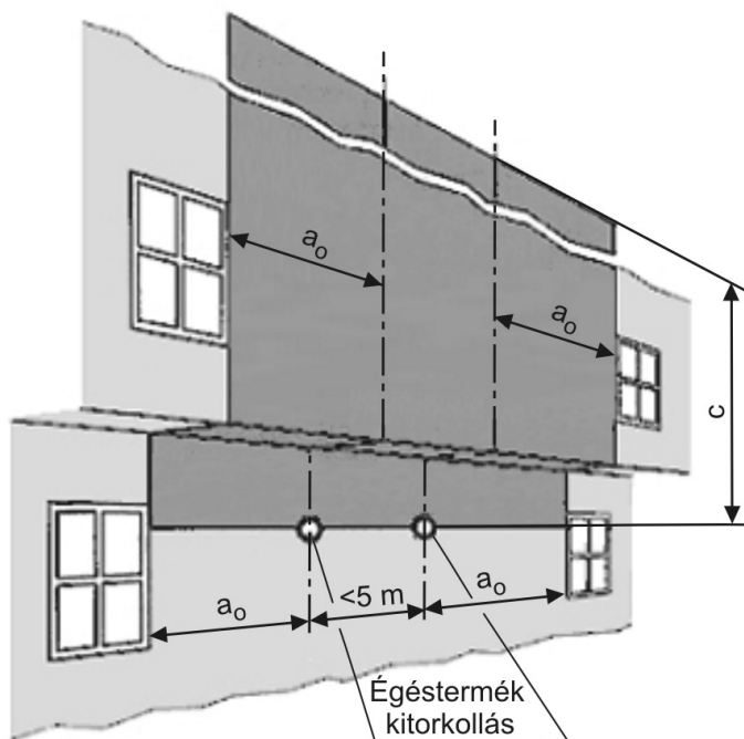
IV.-7. sz. ábra Kétszeres égéstermék-kitorkollások legkisebb távolsága nyitható ablakoktól vagy homlokzati ajtóktól előreugró homlokzatok esetén
