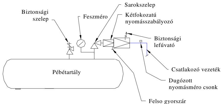
III.-8. sz. ábra Példa tartályra szerelt nyomásszabályozó max. 24 [kg/h] gázélvételre
