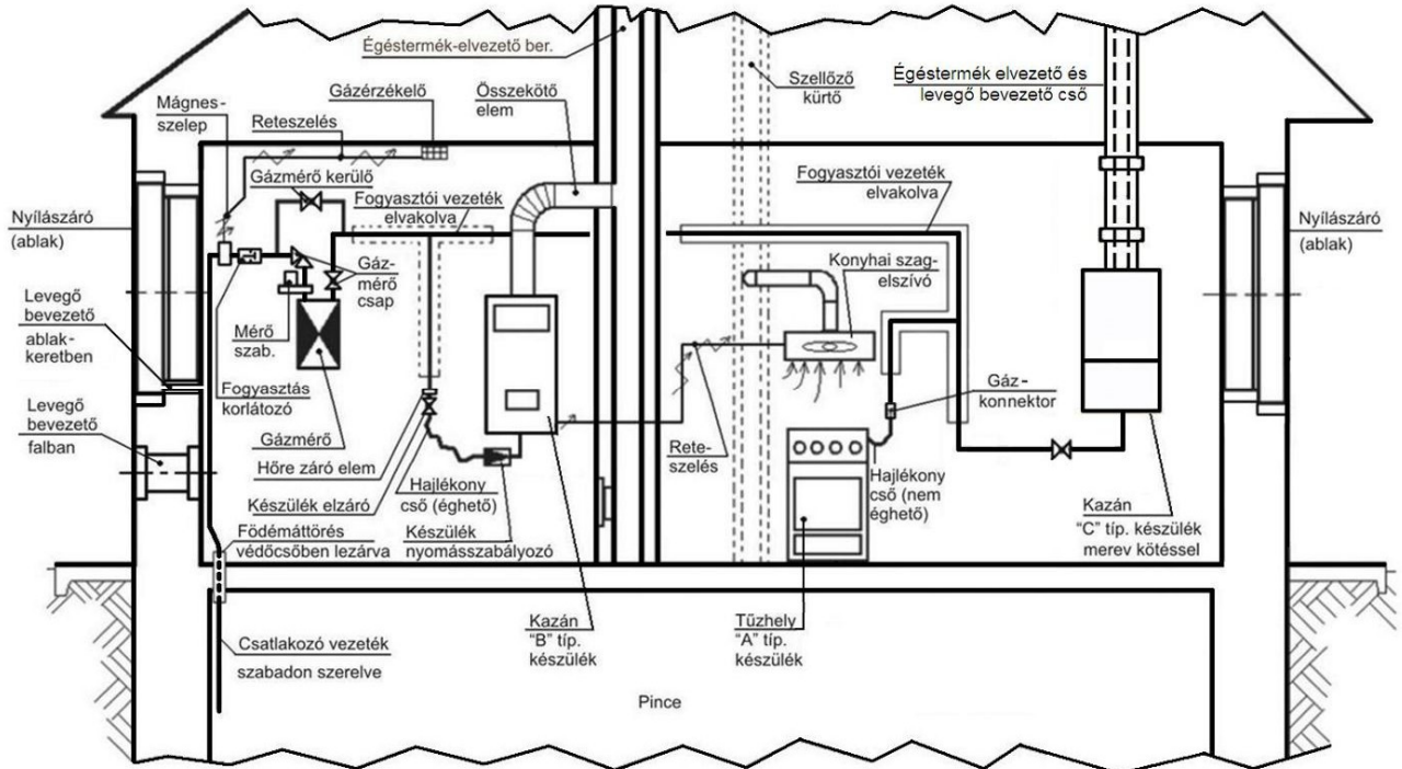
III.-13. sz. ábra A fogyasztói berendezés lehetséges szerelvényei és tartozékai
