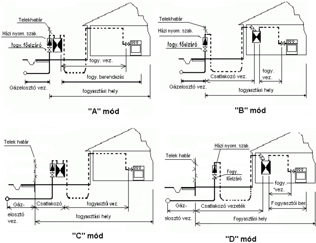
II.-3. sz. ábra Közép, vagy nagyközép nyomású vezetékről ellátott fogyasztói berendezések előkertes beépítés esetén
