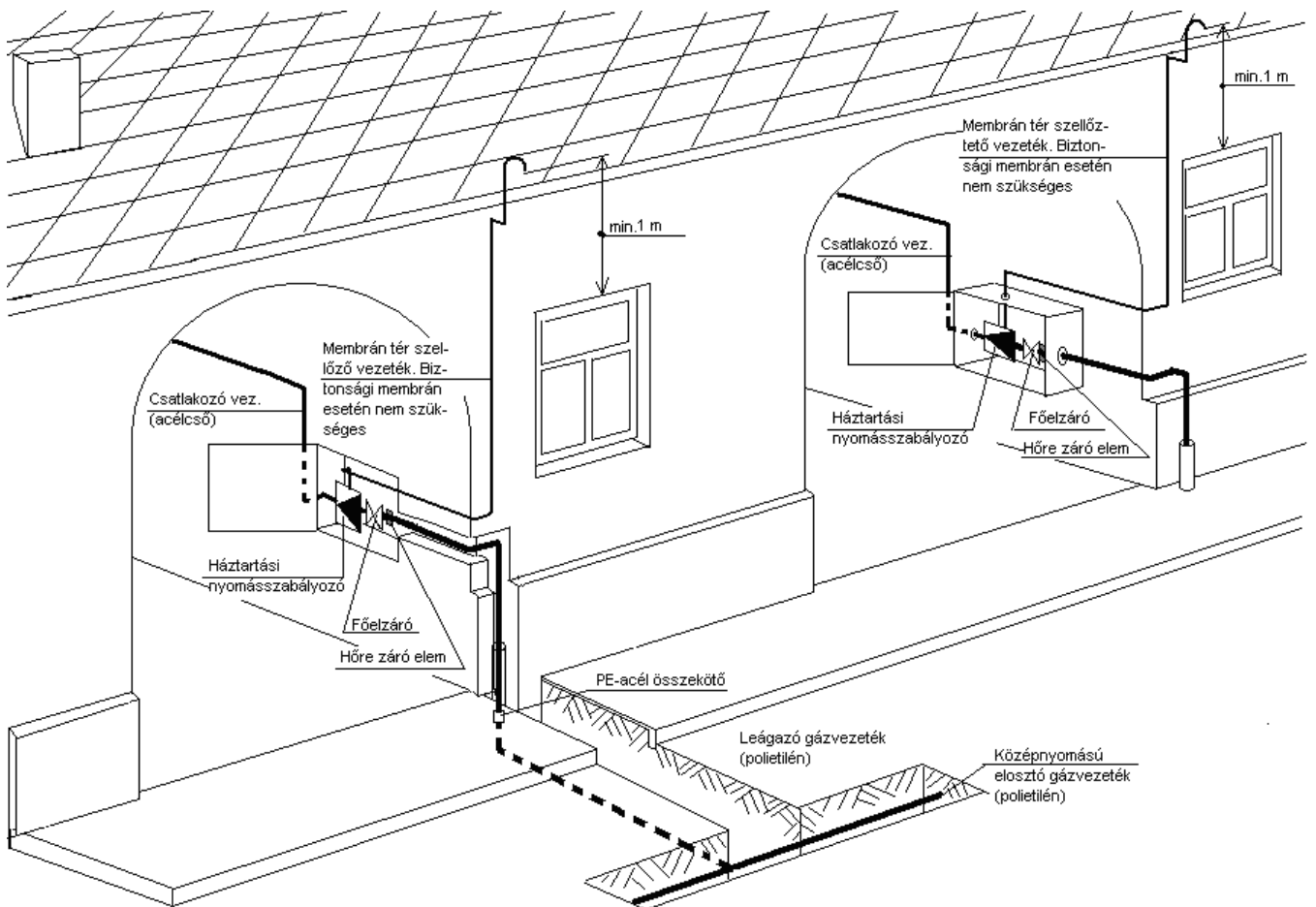
III.-4. sz. ábra Kapualjban elhelyezett házi nyomásszabályozó
