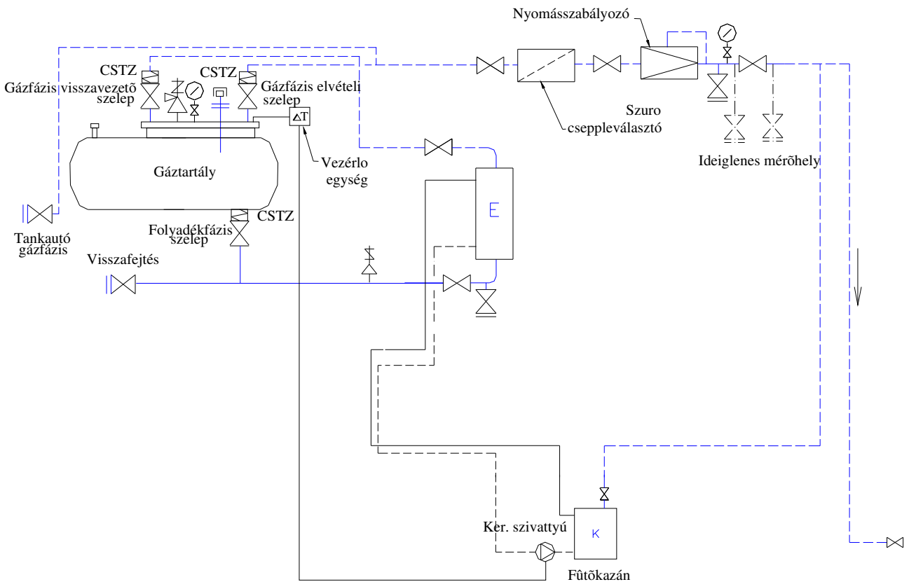
III.-10. sz. ábra Tartályra dolgozó elpárologtató szokásos beépítése
