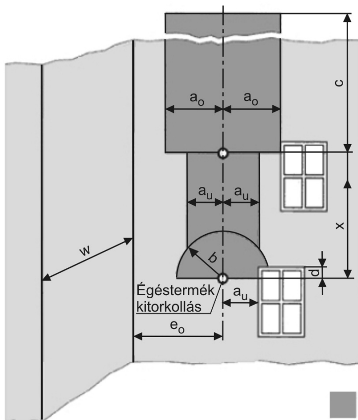
IV.-8. sz. ábra Kétszeres égéstermék-kitorkollások legkisebb távolsága nyitható ablakoktól vagy homlokzati ajtóktól sarkos elhelyezkedésű homlokzatoknál, ablak nélküli haránthomlokzat esetén
